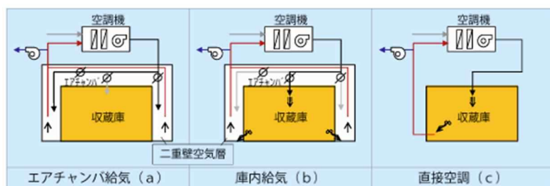
図 4 収蔵庫の空調方式
