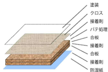
図 5 クロス貼り合板の構成
