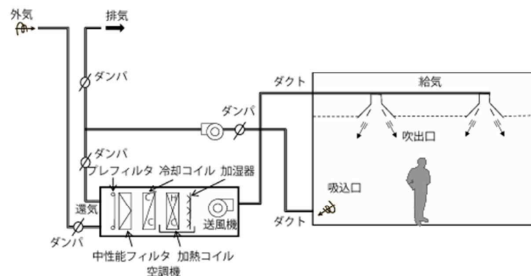
図 3 空調のしくみ
