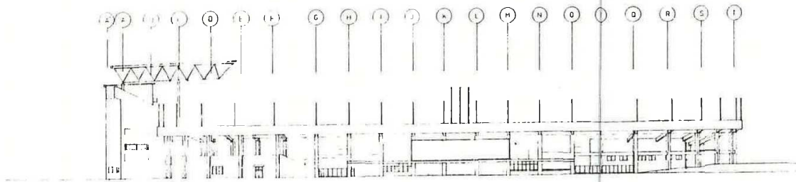
图 4 剖面图 (1:200 1/3)
