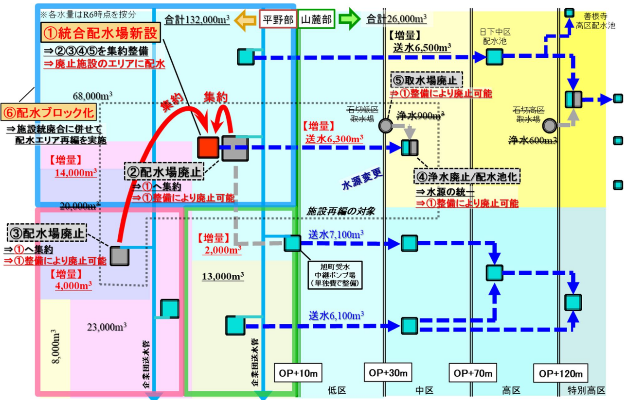
図 4.6 水道施設再編事業の計画概要（上図）及び給水区域モデル・水運用フロー（下図）
