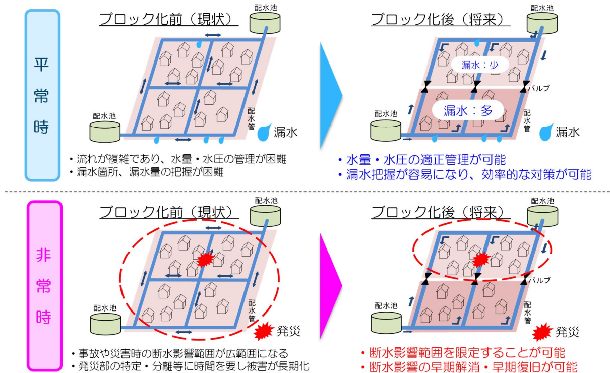
図 4.5 配水ブロック化による効果
