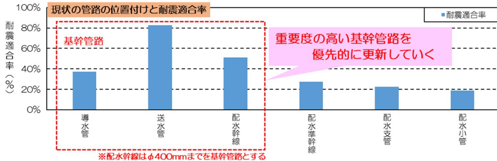
図 4.9 管路の耐震性
