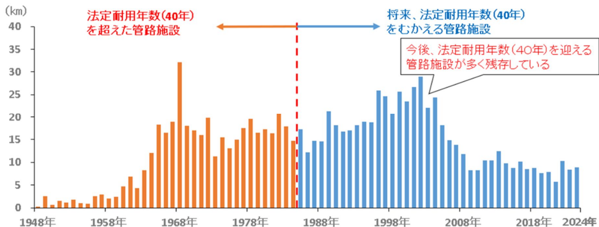
図 4.7 年度別の管路布設延長
