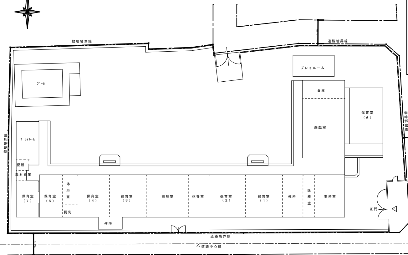
配置図 1 : 2 0 0
