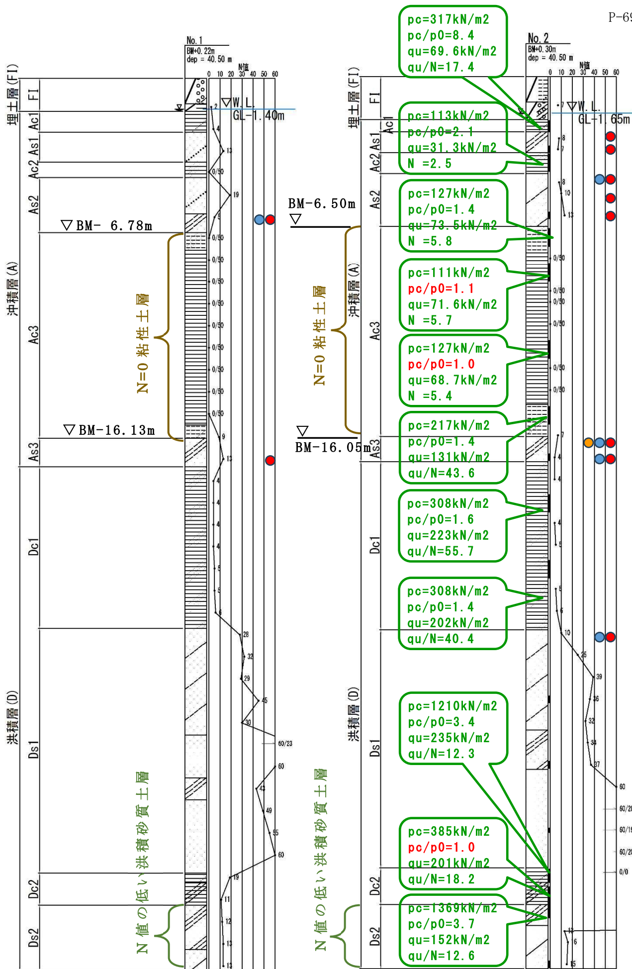
図 6.1-1 調査結果概略図 《別添資料2 地質調査結果》 p.130
