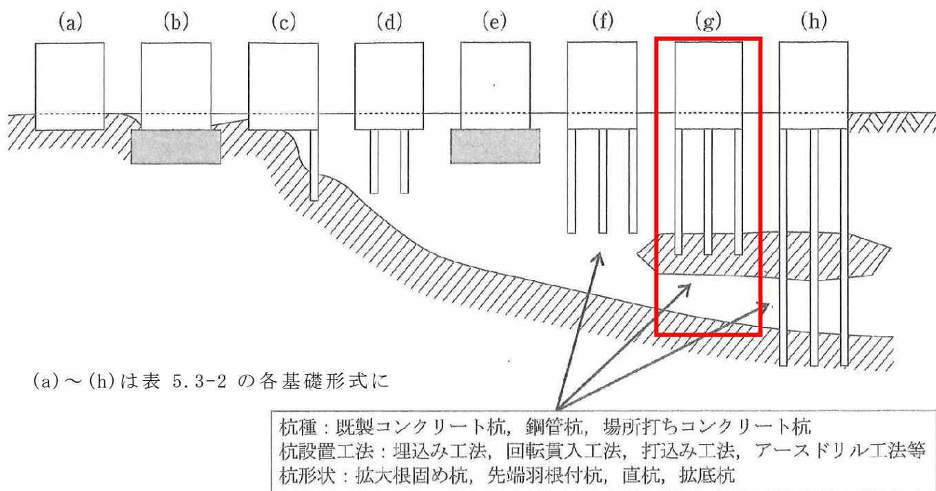
図 5.3-1 支持地盤の深度と適用可能な基礎形式（建築基礎構造設計指針 2019 年版）
