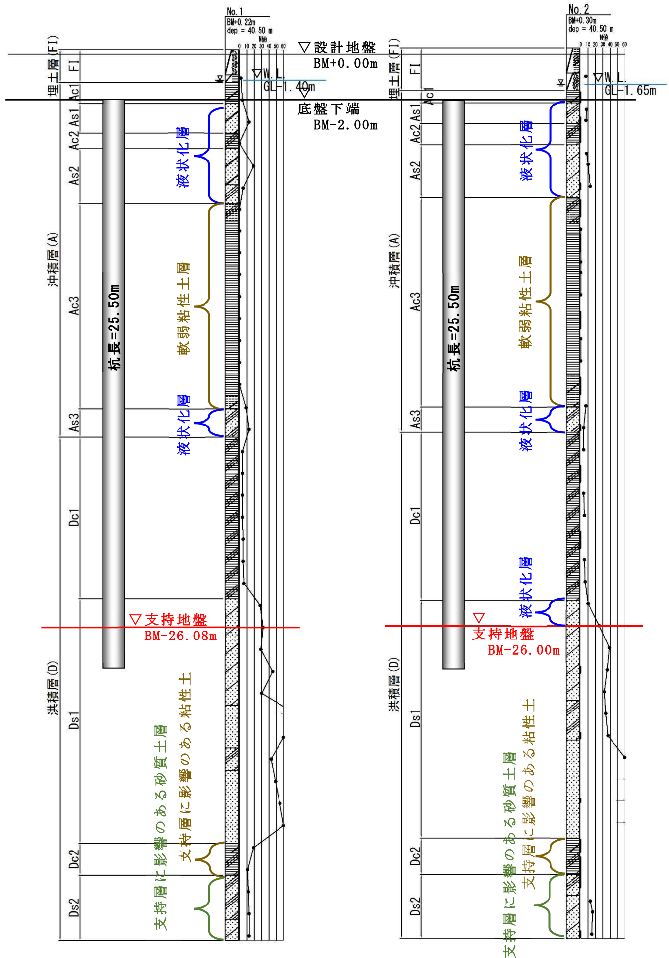
図 5.3-2 支持地盤提案図 《別添資料2 地質調査結果》 p.128
