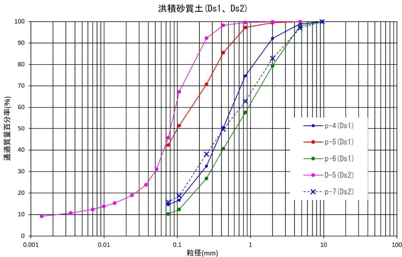
図 4.4-2 粒径加積曲線
