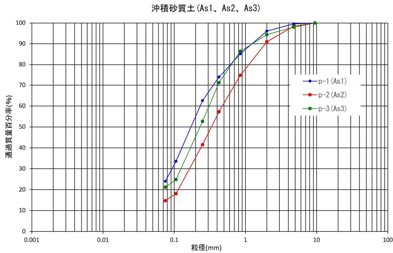
図 4.4-1 粒径加積曲線
