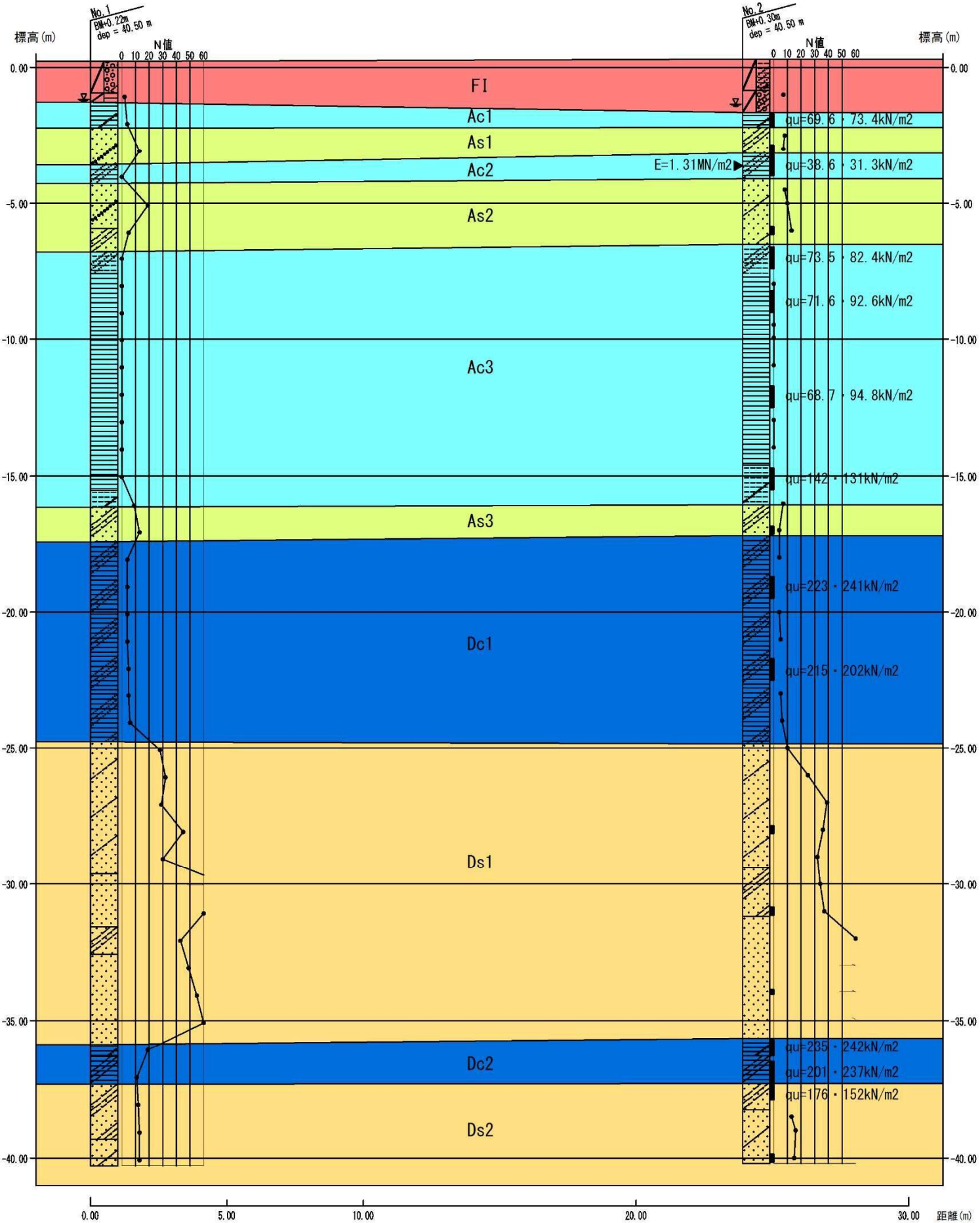
図 4.1-3 推定地質断面図
