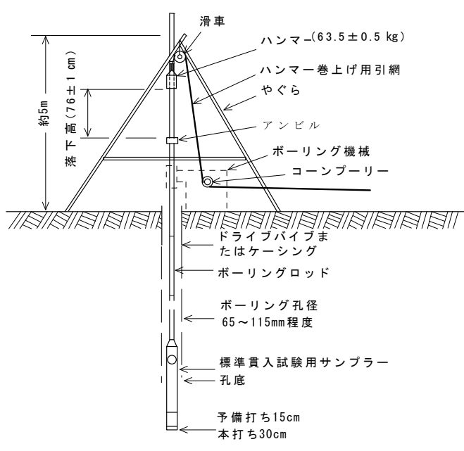
標準貫入試験模式図
