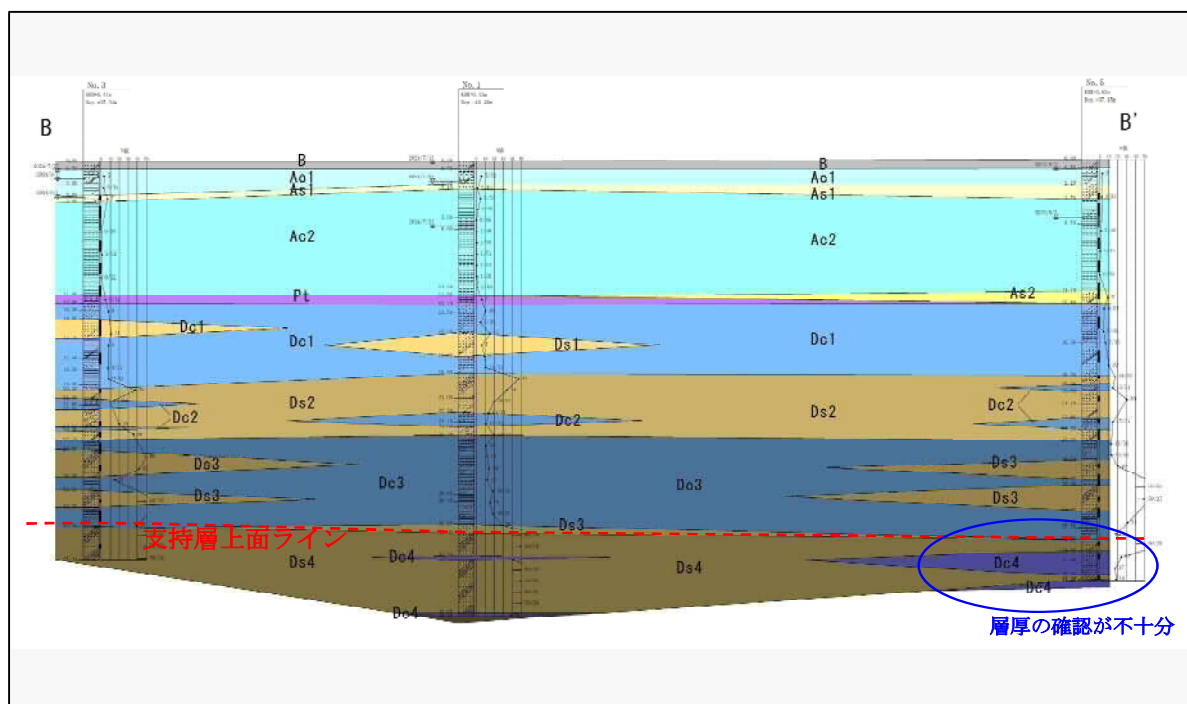
図 5.2.1 支持層の検討(図 5.1.3 に加筆)
