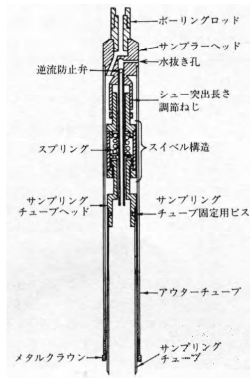
図 2.4.2 ロータリー式二重管サンプラー
