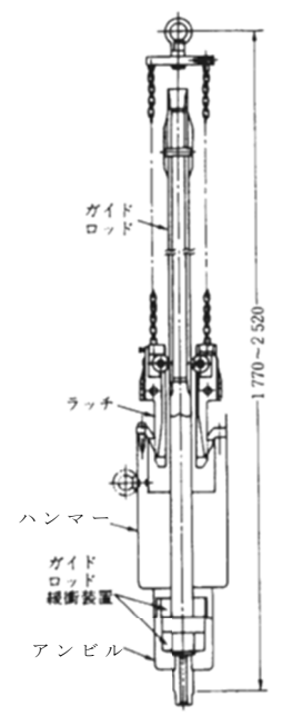
自動落下装置
