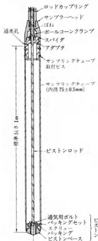
図 2.4.1 シンウォールサンプラー
