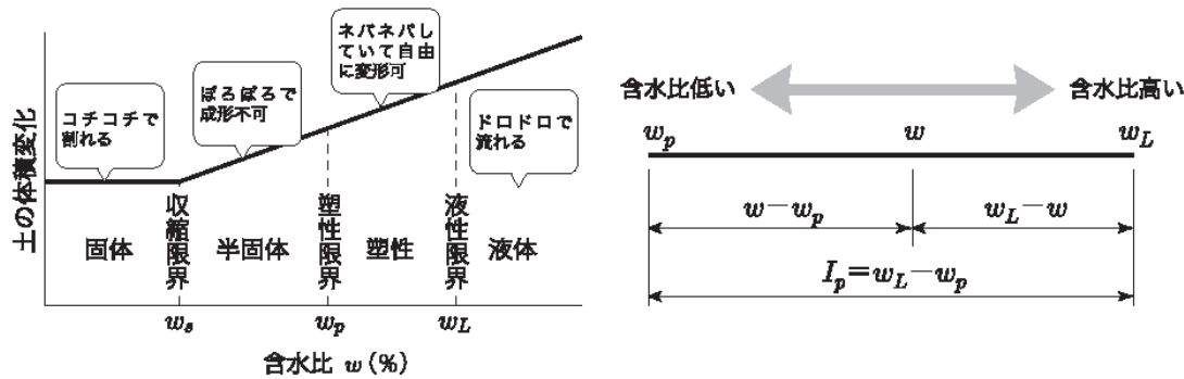
図 4.4-3 土の状態とコンシステンシー限界
