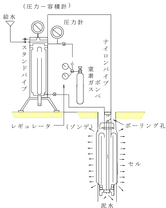
図 3.4-1 孔内水平載荷試験装置概略図
