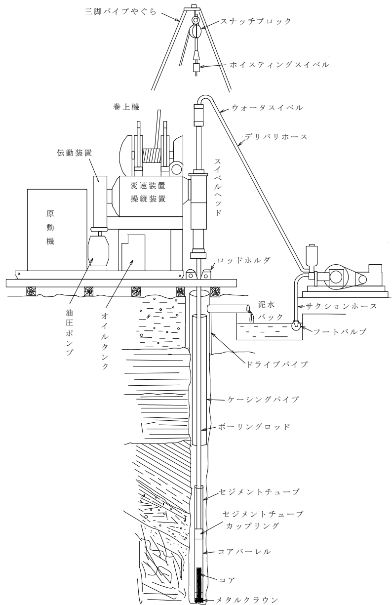
図 3.1-1 ボーリング装置概念図
