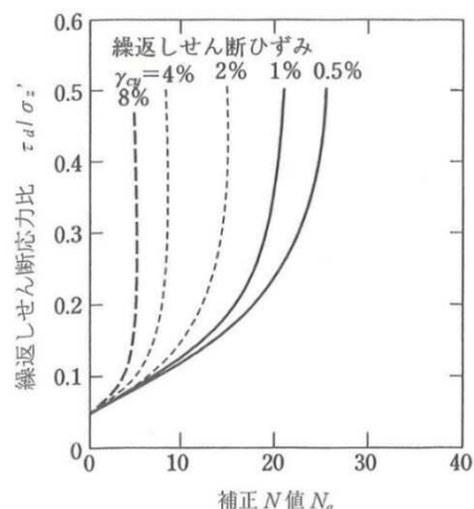
図 5.1-2 補正 N 値と繰返しせん断ひずみの関係
