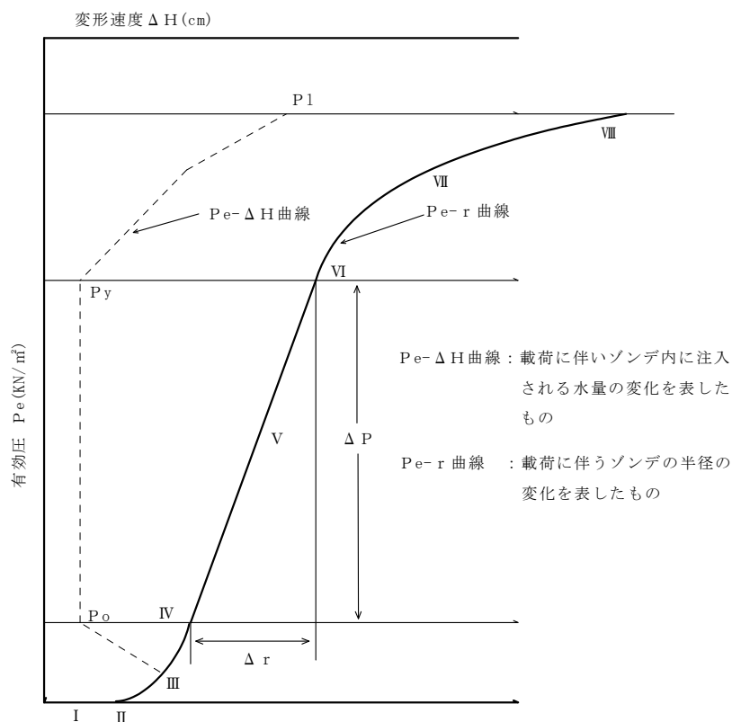
図3.4-2 孔内水平载荷試験結果の解析模式図
