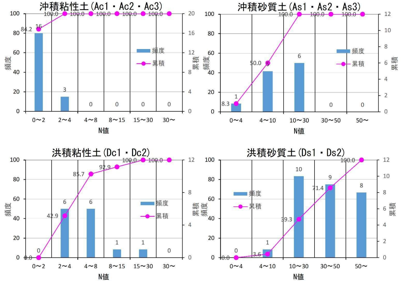
図 4.2-1 標準貫入試験結果図
