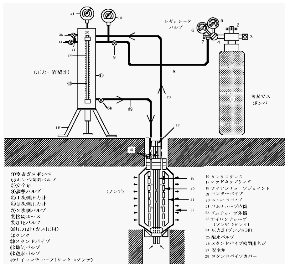
図 2.3.1 試験器具概略図
