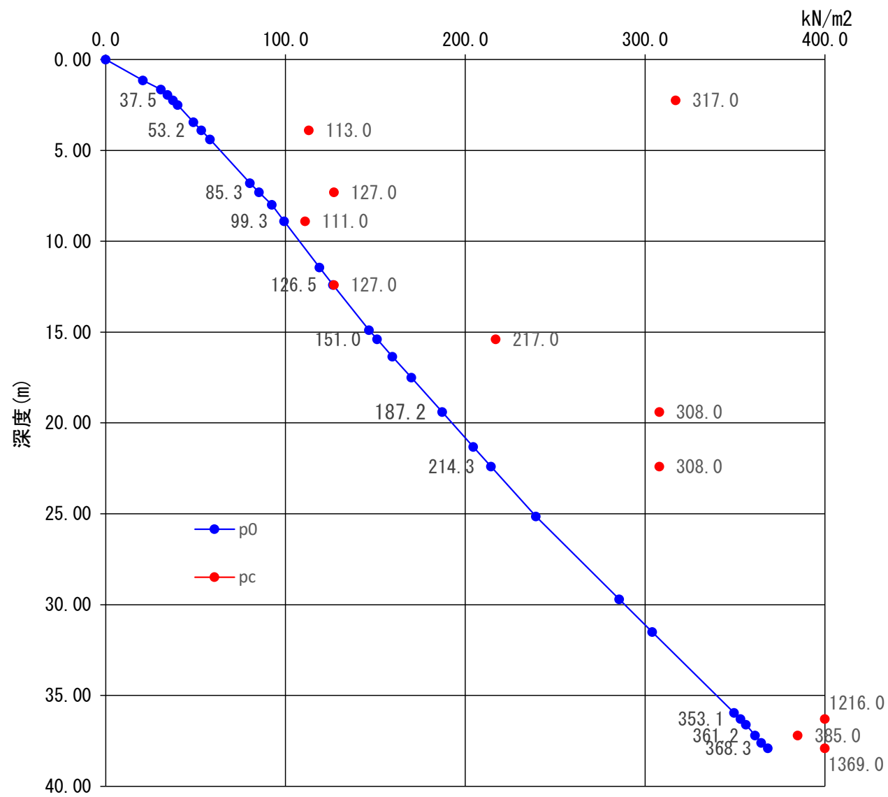
図 4.4-5 圧密降伏応力度と有効土被り圧関係図
