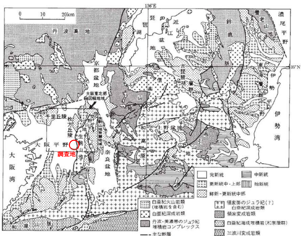
図 3.2.1 近畿・東海地方の地質概略図
