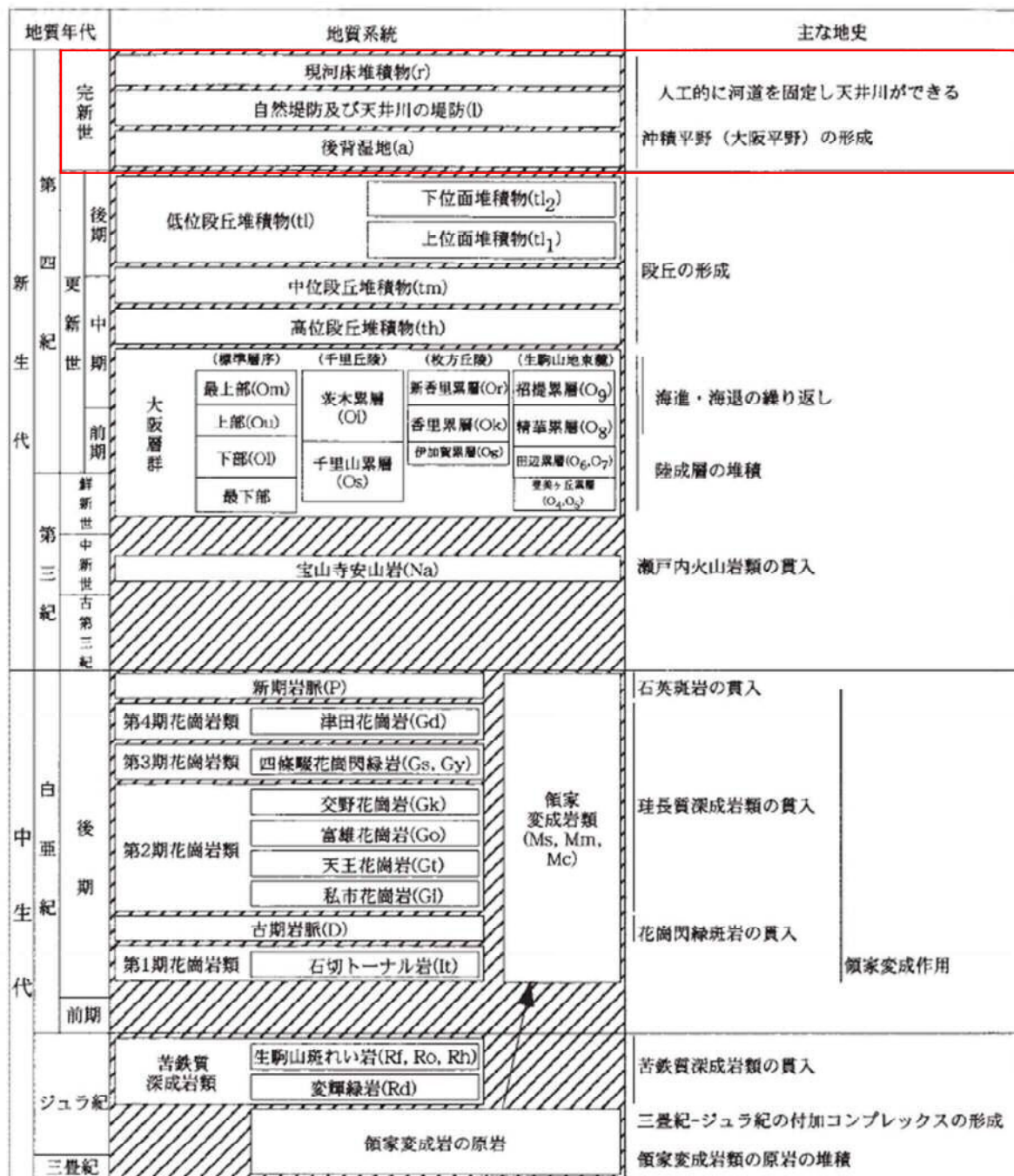
図 3.2.2 調査地周辺地域の層序総括図
