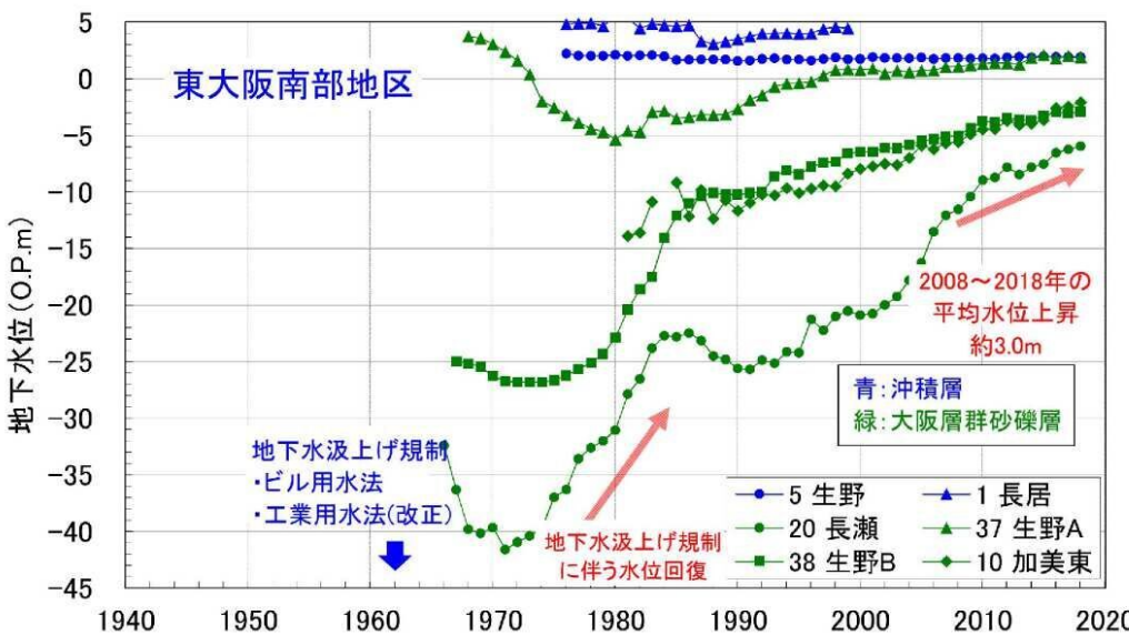
図 4.1-2 地下水観測値(参考)
