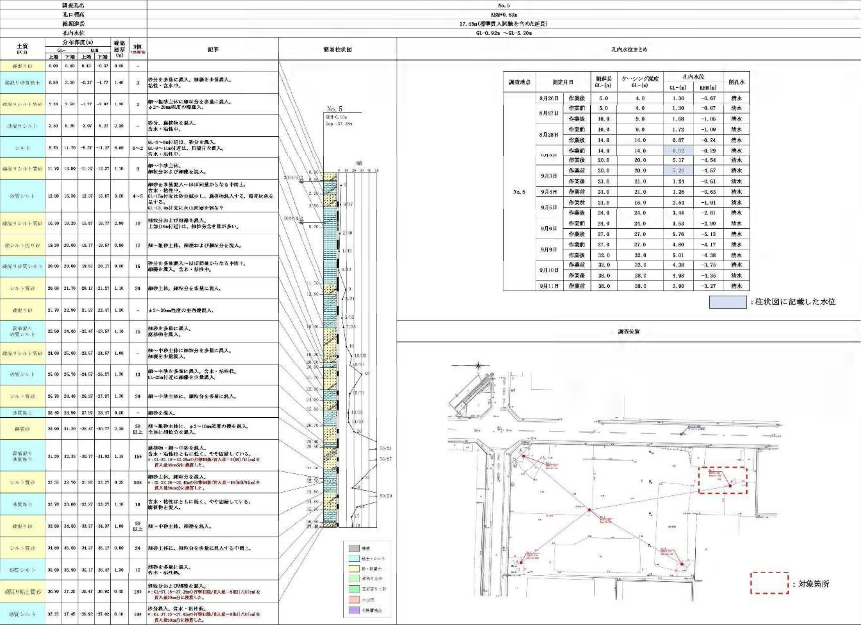
図 4.1.5 ボーリング概要図(No.5)
