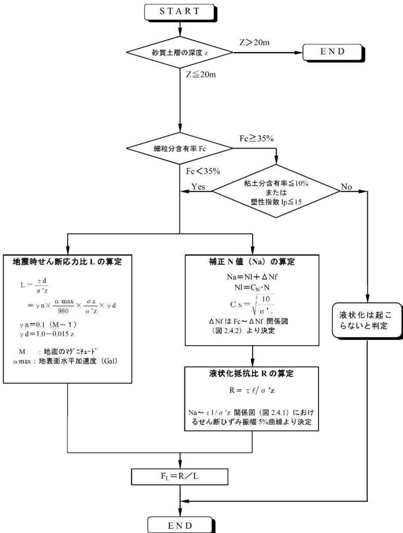
図 5.1-1 液化化判定手順 (FL 法) (液化化判定プログラムマニュアル フリーソフト: 中央開発株式会社)
