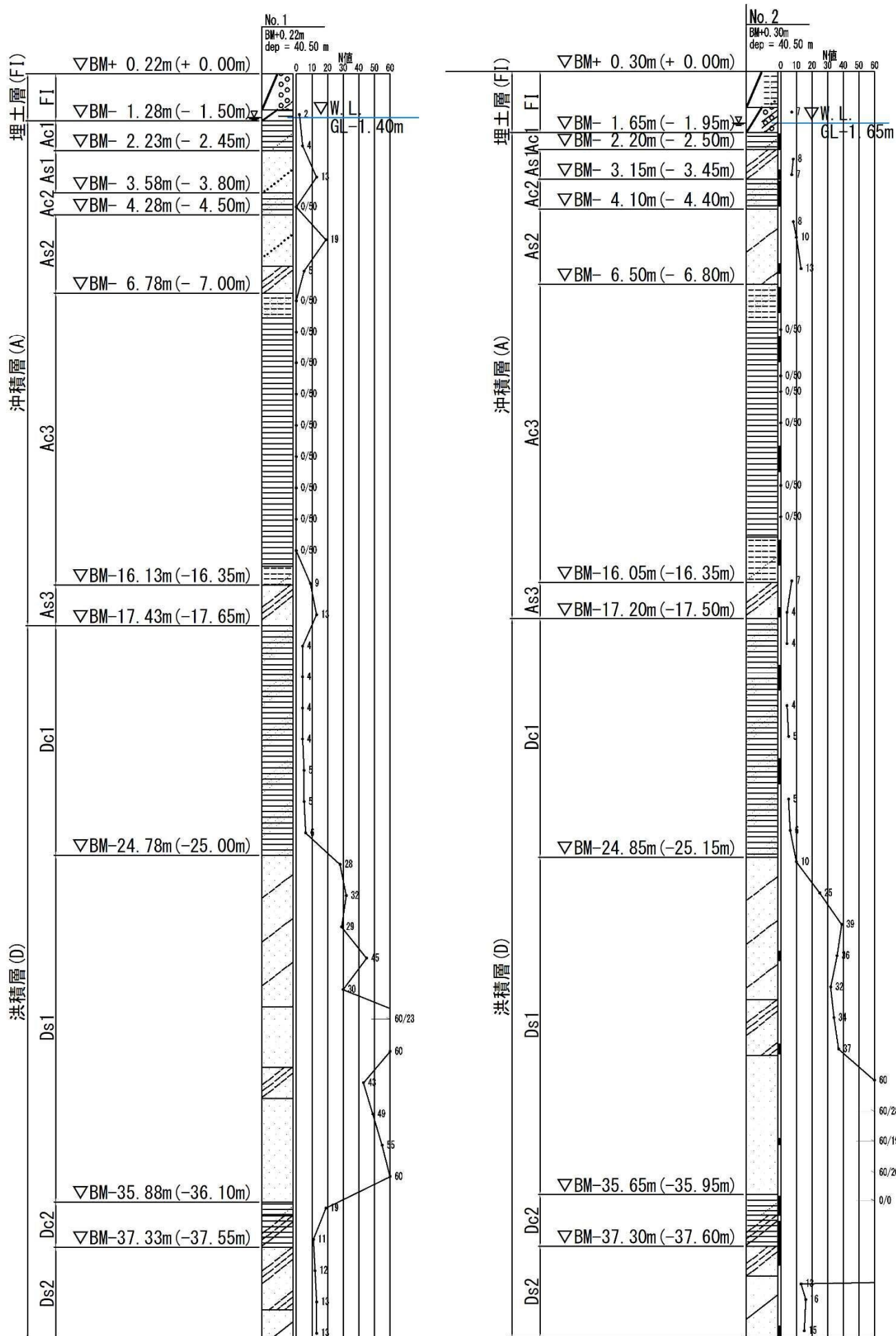
図 4.1-1 土層構成図 《別添資料2 地質調査結果》 p.86
