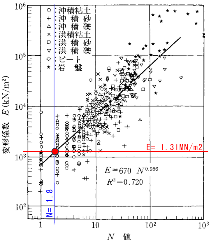
図 4.3-1 N 値と変形係数 E 関係図 (地盤調査の方法と解説 地盤工学会)
