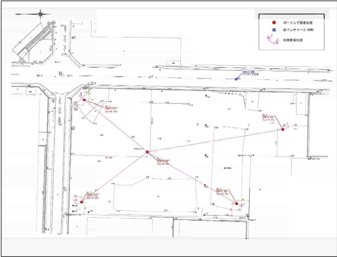
図 5.1.1 断面位置図
