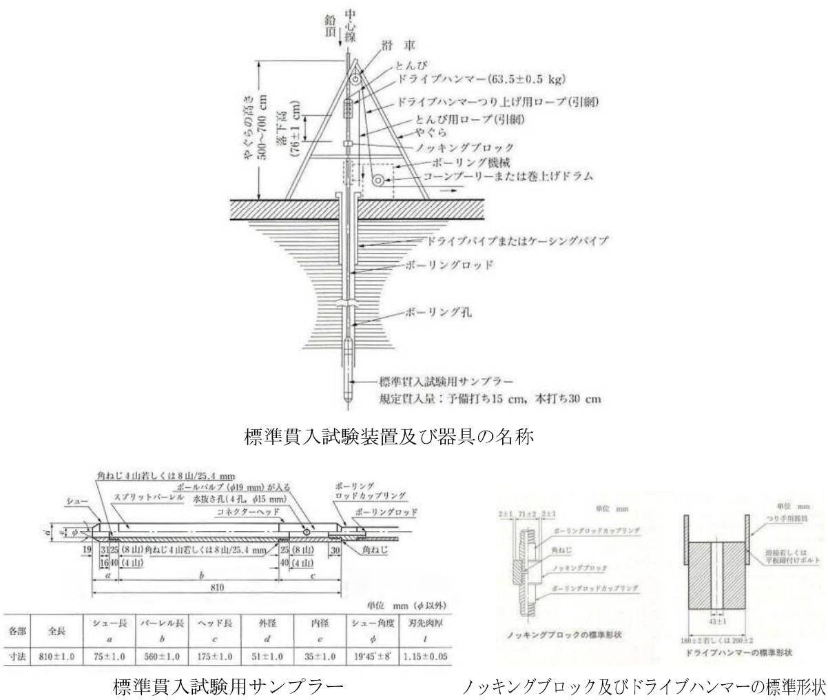
図 2.2.1 標準貫入試験概念図
