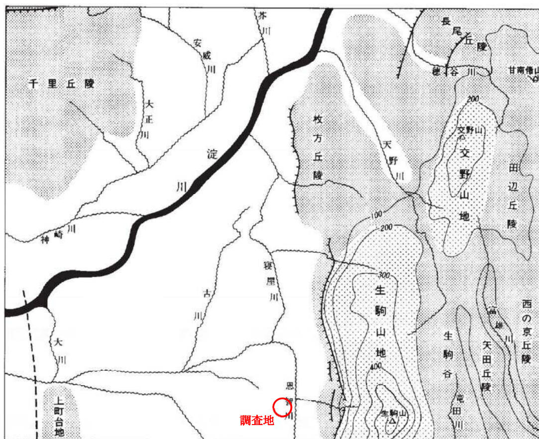
図 3.1.1 調査地周辺の地形区分
