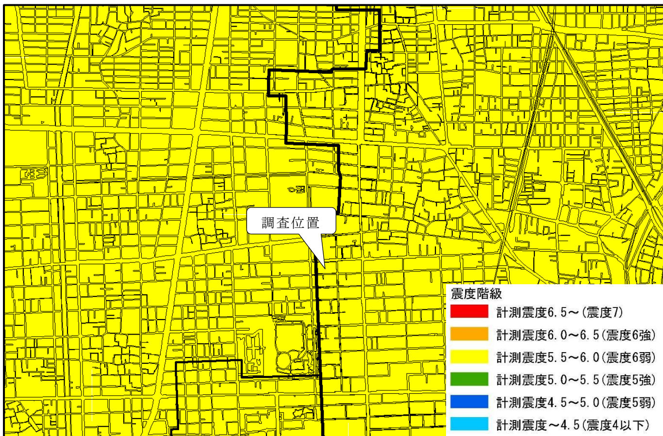
図 5.1-4 調査地周辺の震度分布図(大阪府 HP 参照)
