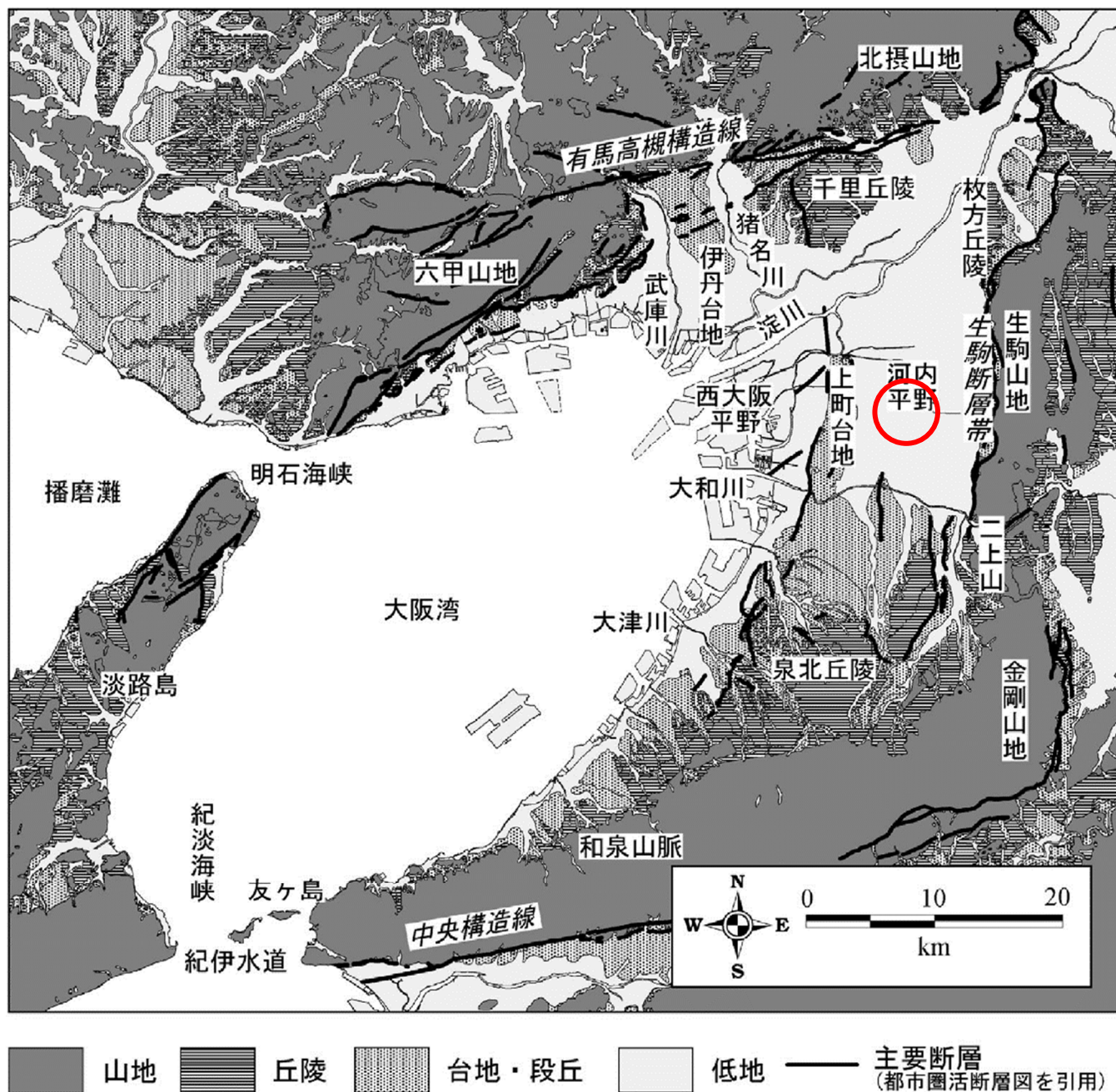
図 2.1-1 調査地周辺地形分類図（新関西地盤 2007 年版より抜粋） ○：調査位置
