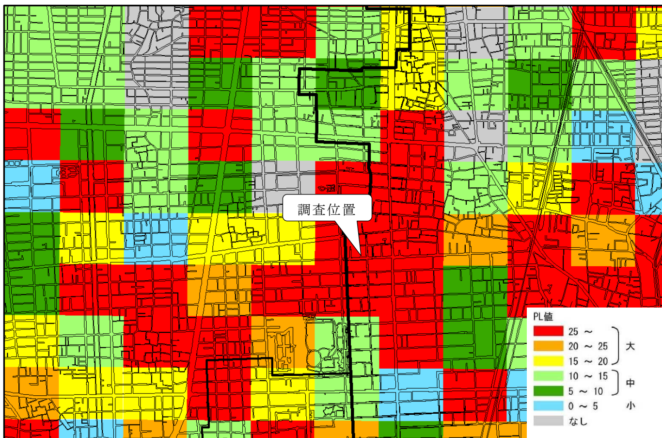
図 5.1-3 調査地周辺の液状化ハザードマップ(南海トラフの最大クラスの地震：大阪府 HP 参照)
