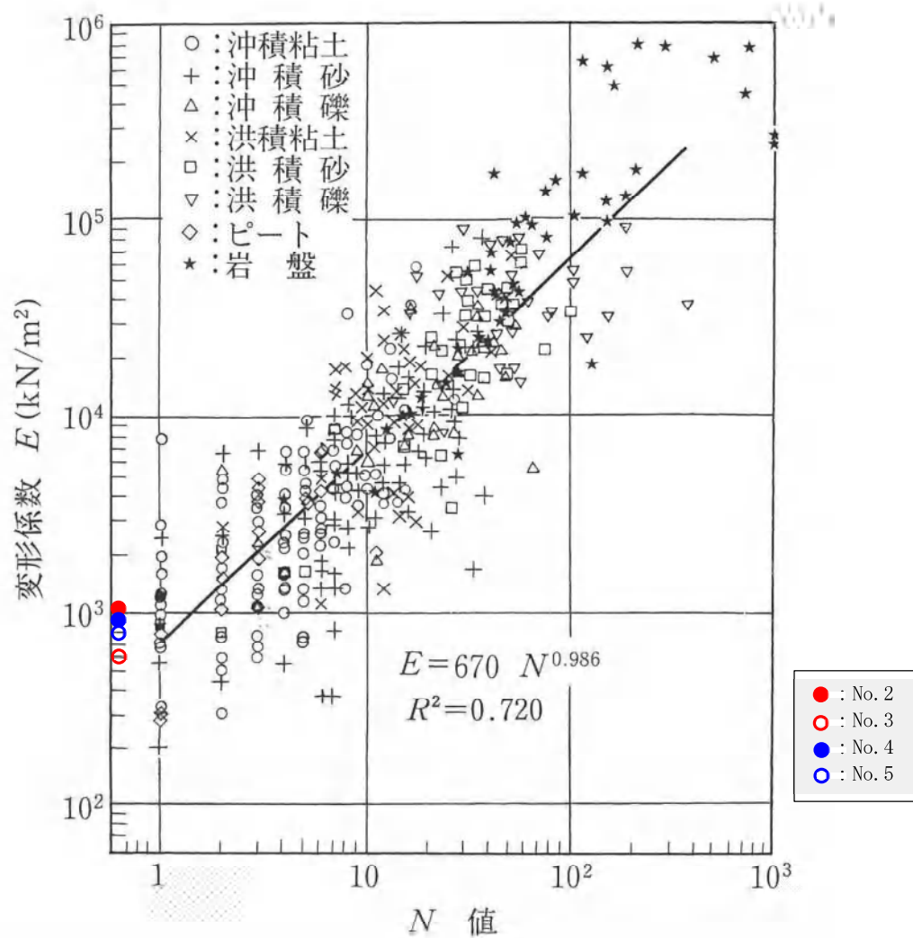
図 4.2.1 孔内载荷試験により得られた変形係数と N 値の関係 (土谷・豊岡に加筆修正)
