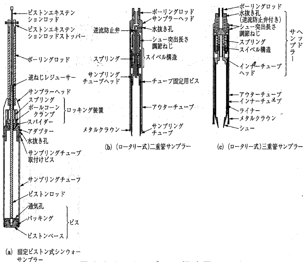
図 3.3-1 サンプラー概略図
