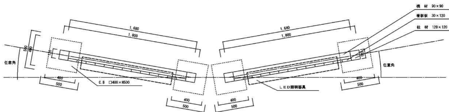
立面図
