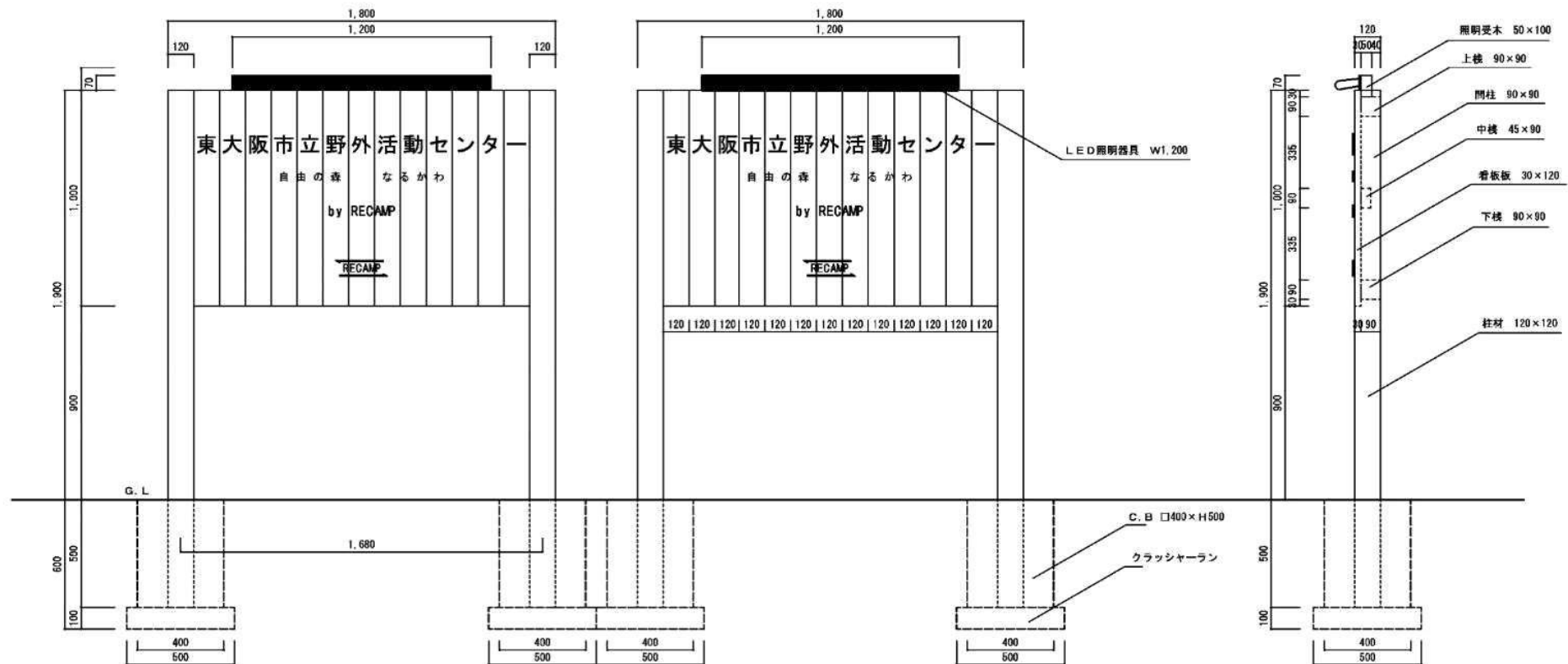
立面図
