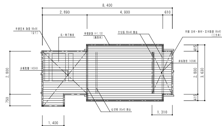
床板割付図 1/100
