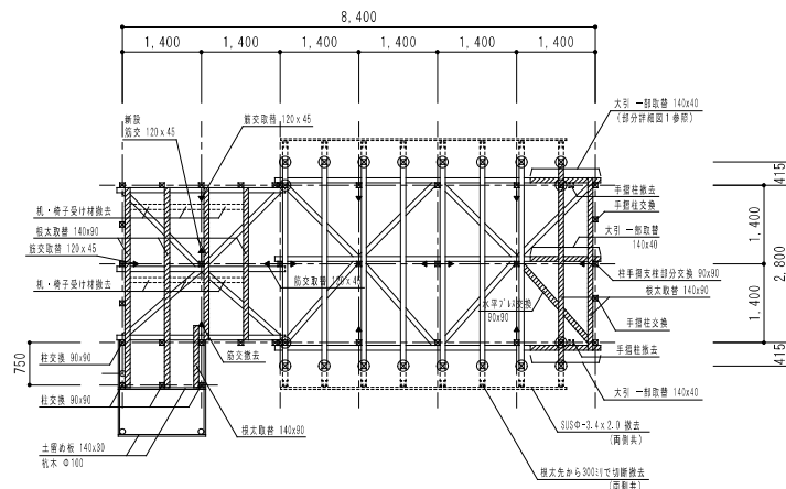
凡例 ⊗ : 手摺支柱 (新設) 90x90 床 伏 図 1/100
