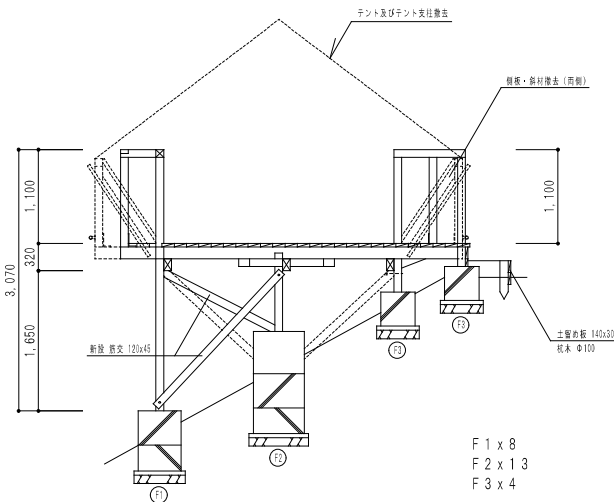
基本断面図 1/60
