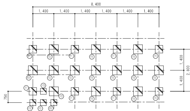
基 礎 図 1/100
