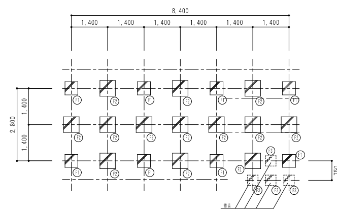
基 礎 図 1/100
