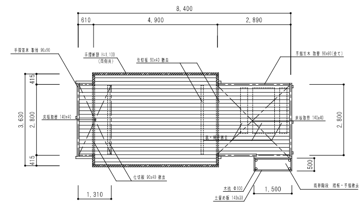
床 板 割 付 図 1/100
