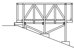
基本立面図 1/100
