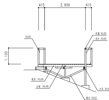
基本断面図 1/100
