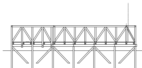
基本立面図 1/100
