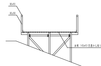
基本断面図 1/100
