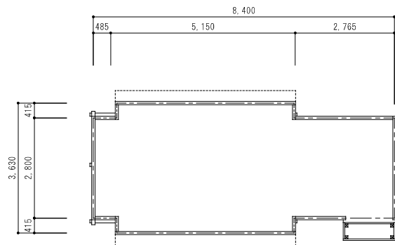
平面図 1/100
