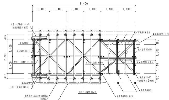
床 伏 図 1/100
