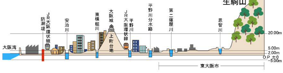
東西断面図(国道308号沿)
