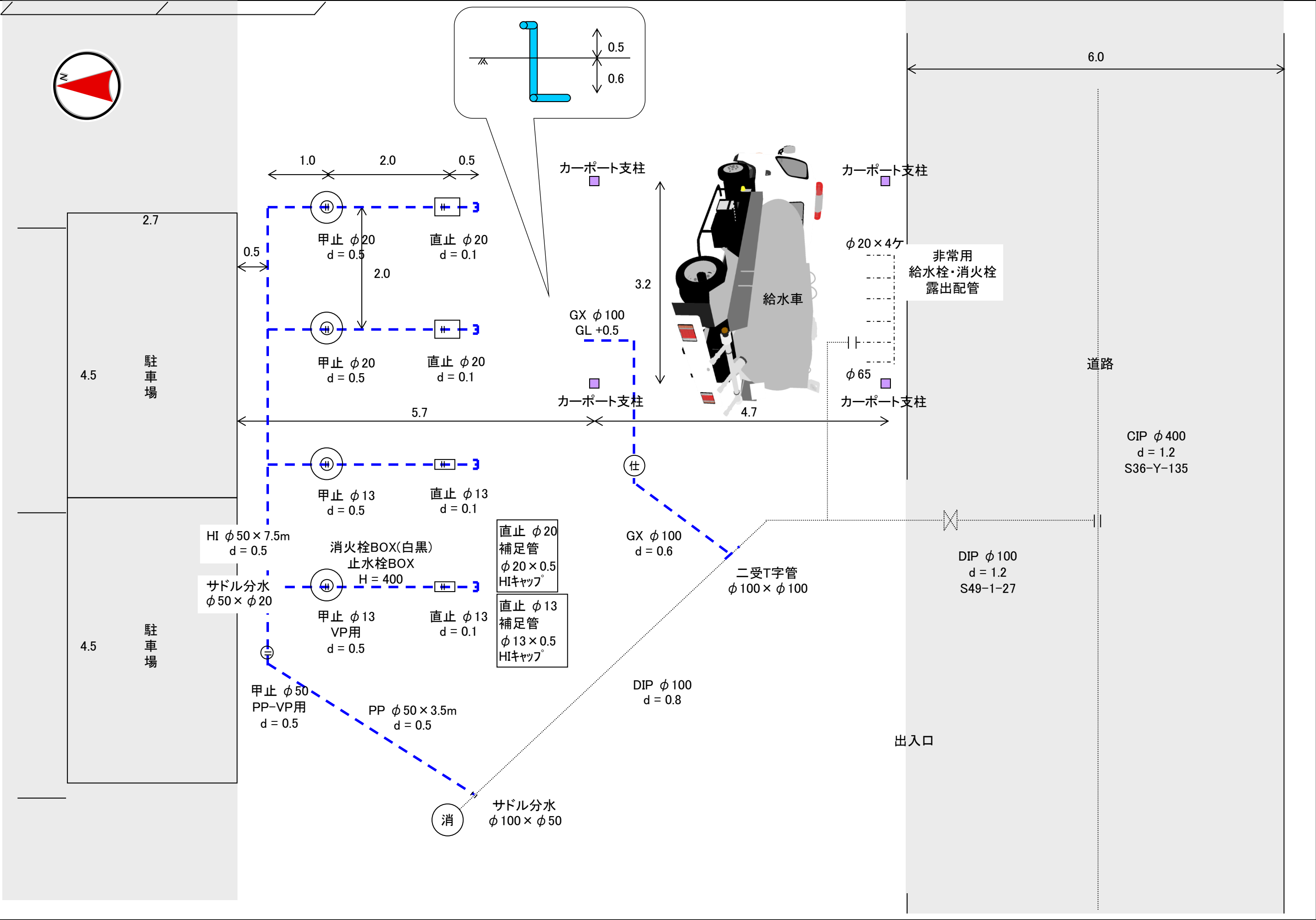
資料22 現水道庁舎の訓練スペース現況図
