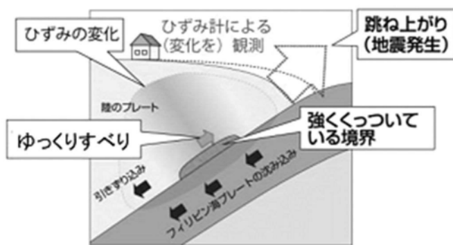
【ゆっくりすべりのイメージ】
