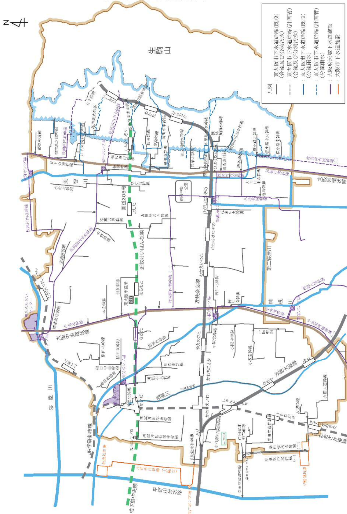
東大阪市下水道幹線図
