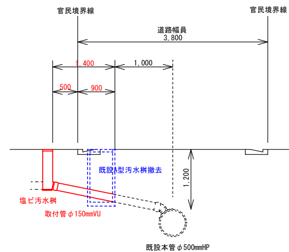
断面図 S=1:50
