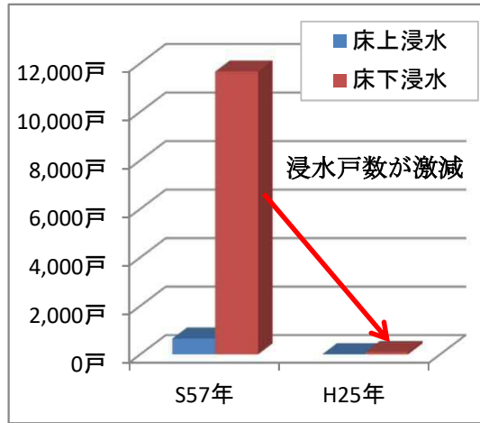
雨水増補管整備 前 浸水状況
