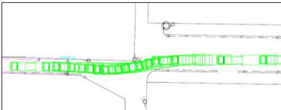
詳細図 B
