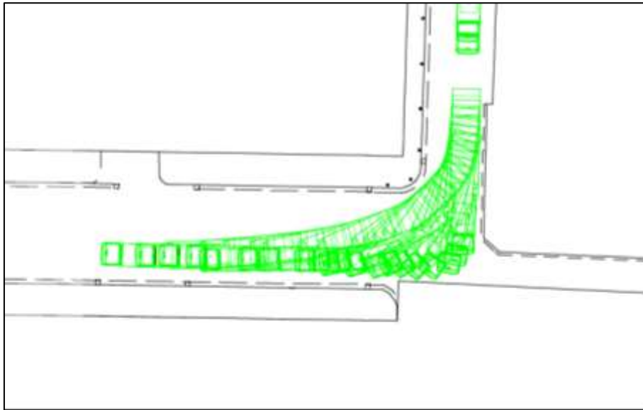
詳細図 A
