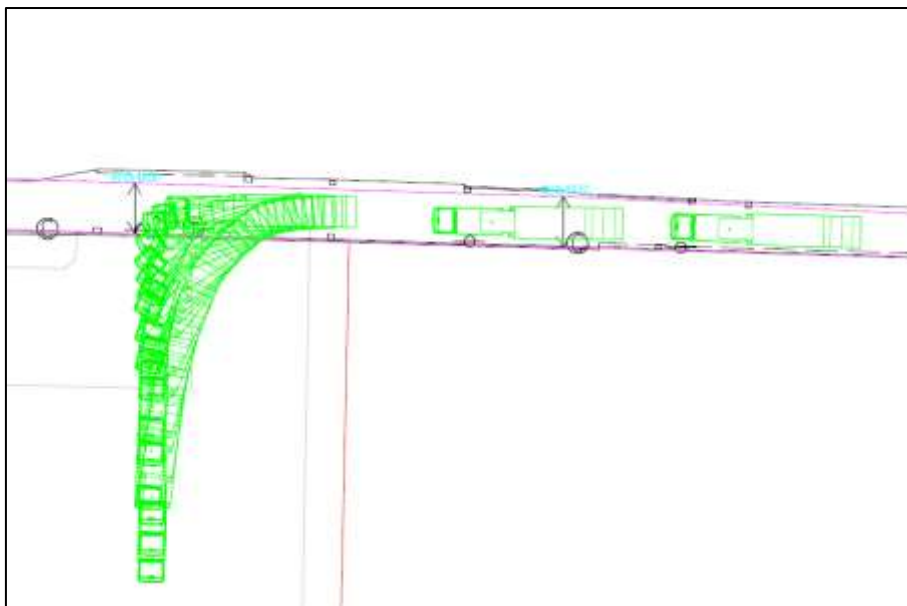
詳細図 C
