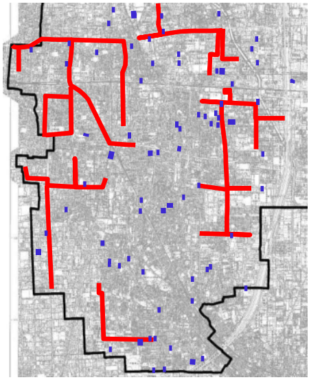
雨水増補管整備 後 浸水状況
