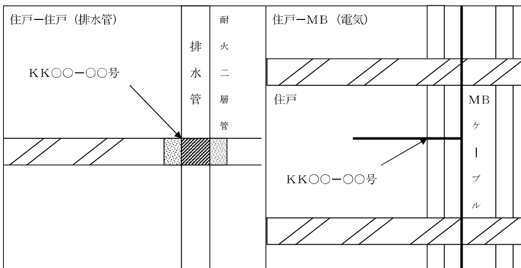
区画貫通処理リスト（詳細図）（例示）
