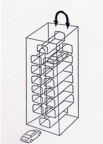
機械式 - 垂直循環方式
