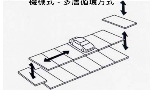
機械式 - 多層循環方式
