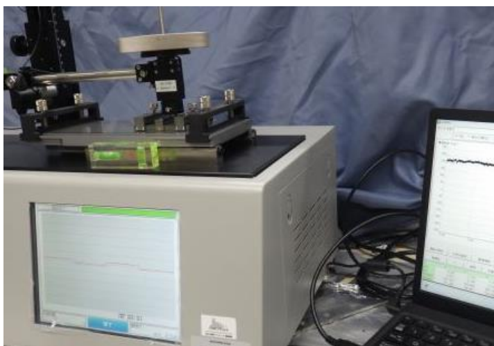
往復摺動式摩擦摩耗試験機
