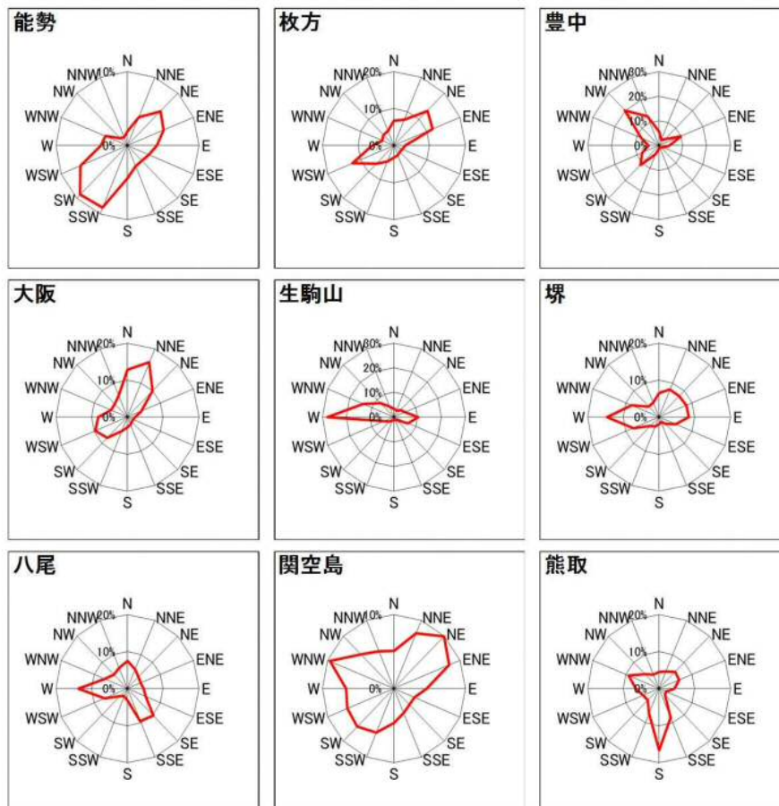
年間の風配図
