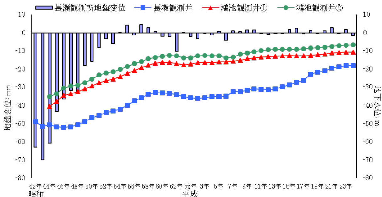
地下水位及び地盤変位の経年変化
