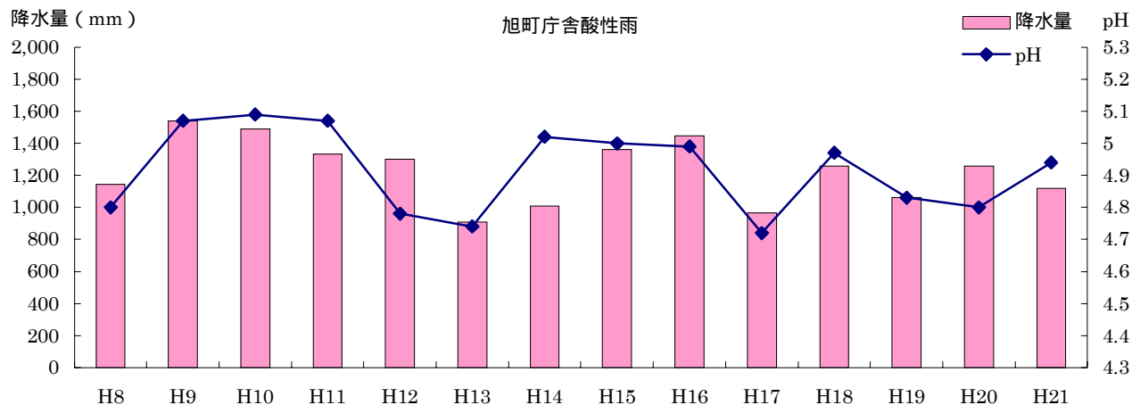
図2-1-20 酸性雨の経年変化
