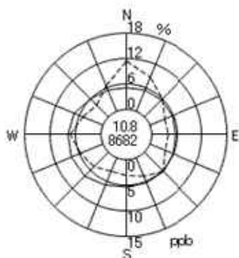
図 2 - 1 - 1 2 一酸化窒素の風向別濃度測定結果
