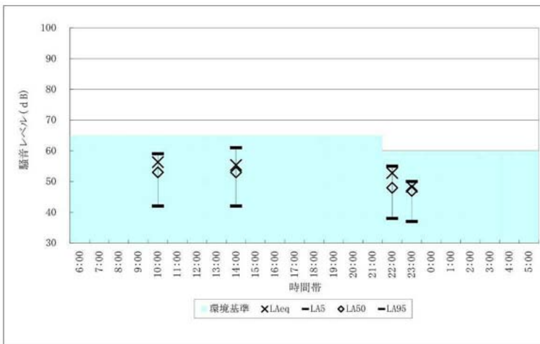
図 2-3-11 騒音測定結果 (No.7:市道東大阪中央線、背後地)
