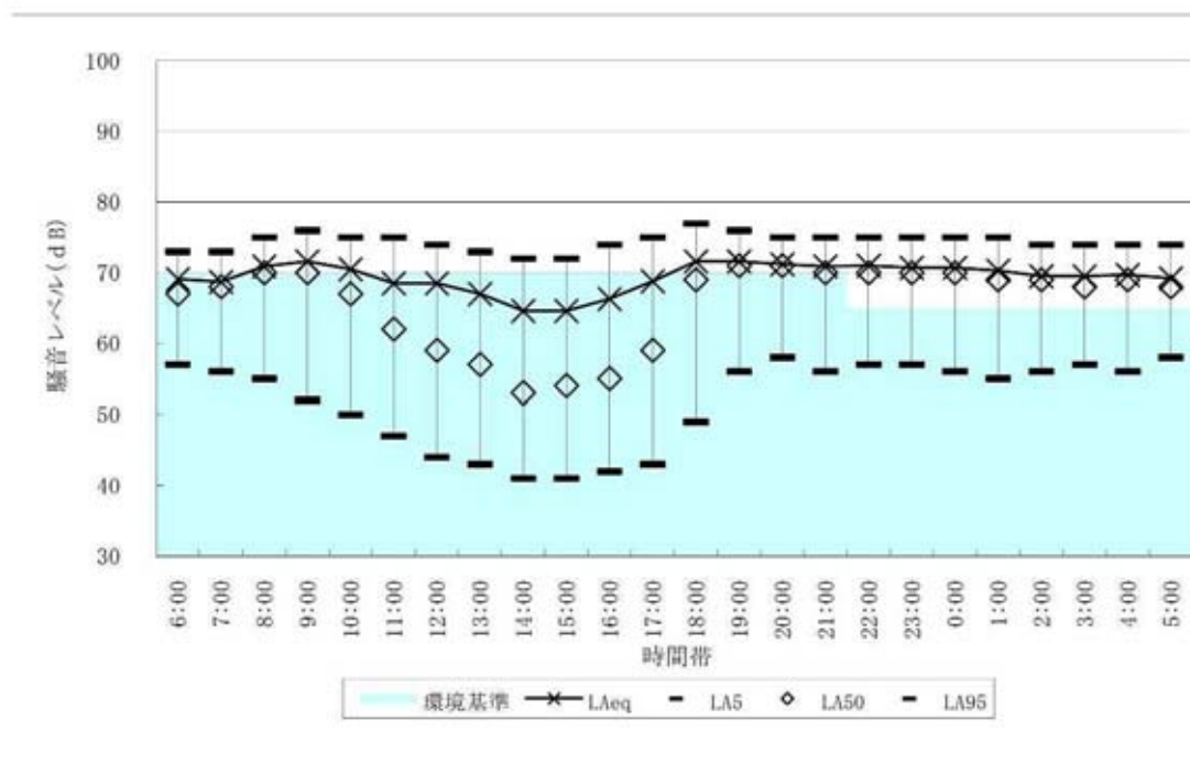
図 2-3-2 騒音測定結果 (No.2:国道 170 号、セリサス番号:1044、沿道)
