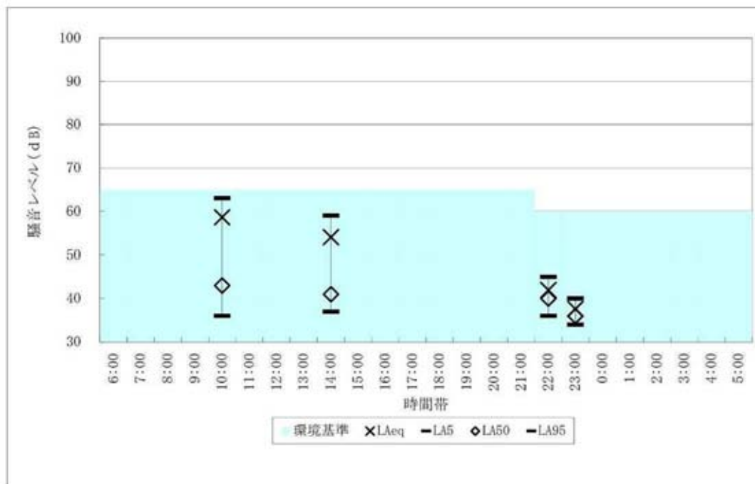
図 2-3-9 騒音測定結果（No.6:市道加納玉串線、背後地）
