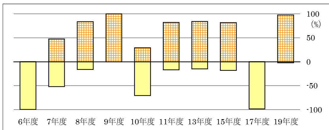
図2-5-2 隆起・沈下測定地点経年変化図
