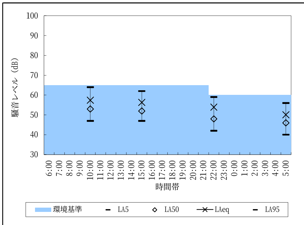
図2-3-7 騒音レベル測定結果（No.5:大阪東大阪線、センサス番号:4136、背後地）
