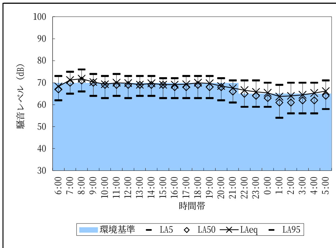
図2-3-3 騒音レベル測定結果（No.3:府道大阪中央環状線、センサス番号:4054、沿道）
