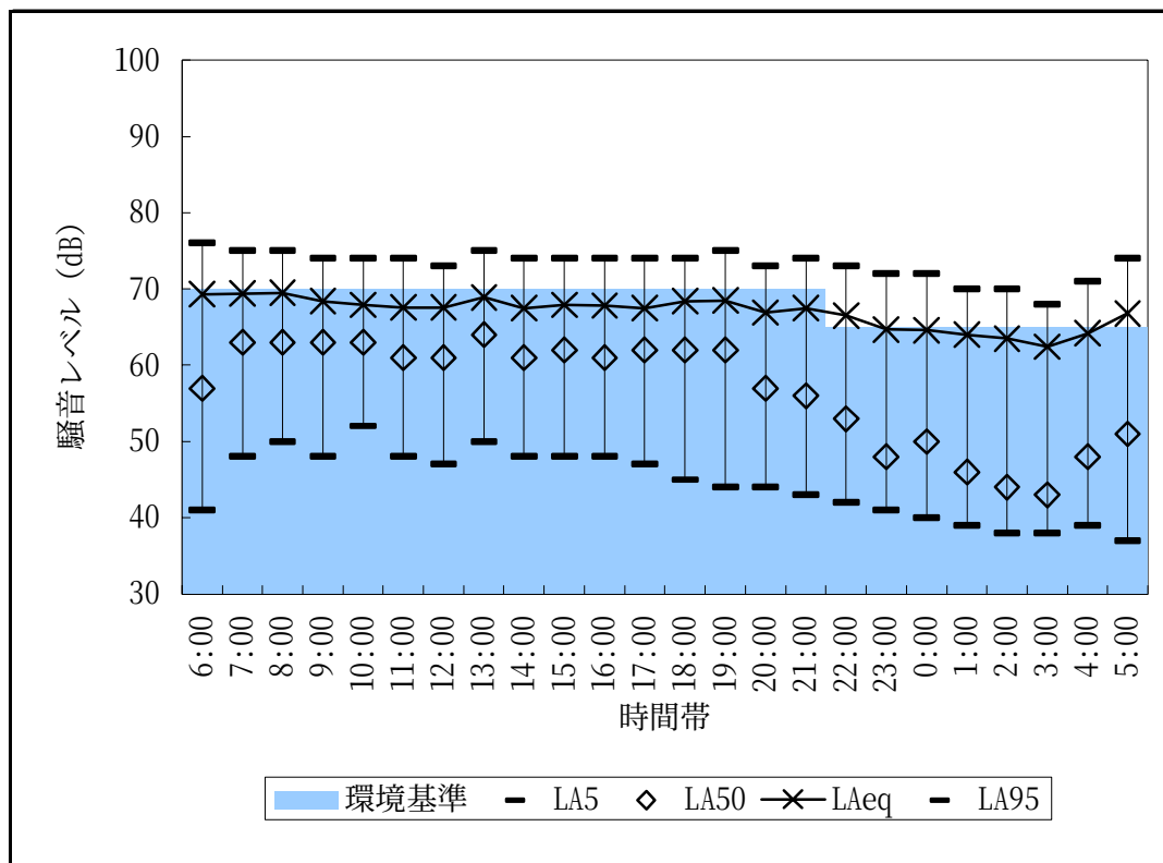
図2-3-10 騒音レベル測定結果（No.7:太平寺寺前線、沿道）
