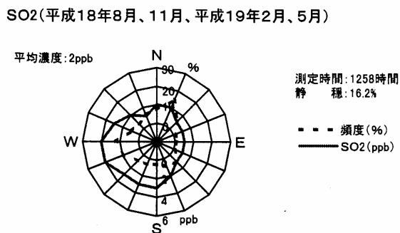
図 2-1-22 二酸化硫黄の風向別濃度測定結果（長田東内介公園）
