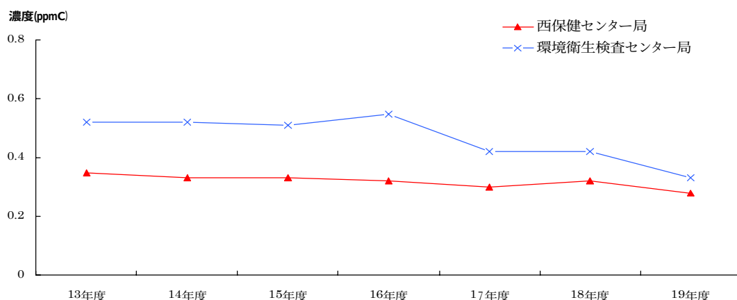
図2-1-5 6～9時における非メタン炭化水素濃度の推移（年平均値）
