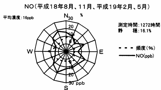
図 2-1-24 一酸化窒素の風向別濃度測定結果 (長田東内介公園)
