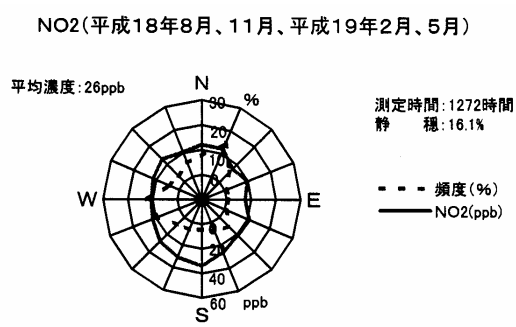
図 2-1-23 二酸化窒素の風向別濃度測定結果（長田東内介公園）
