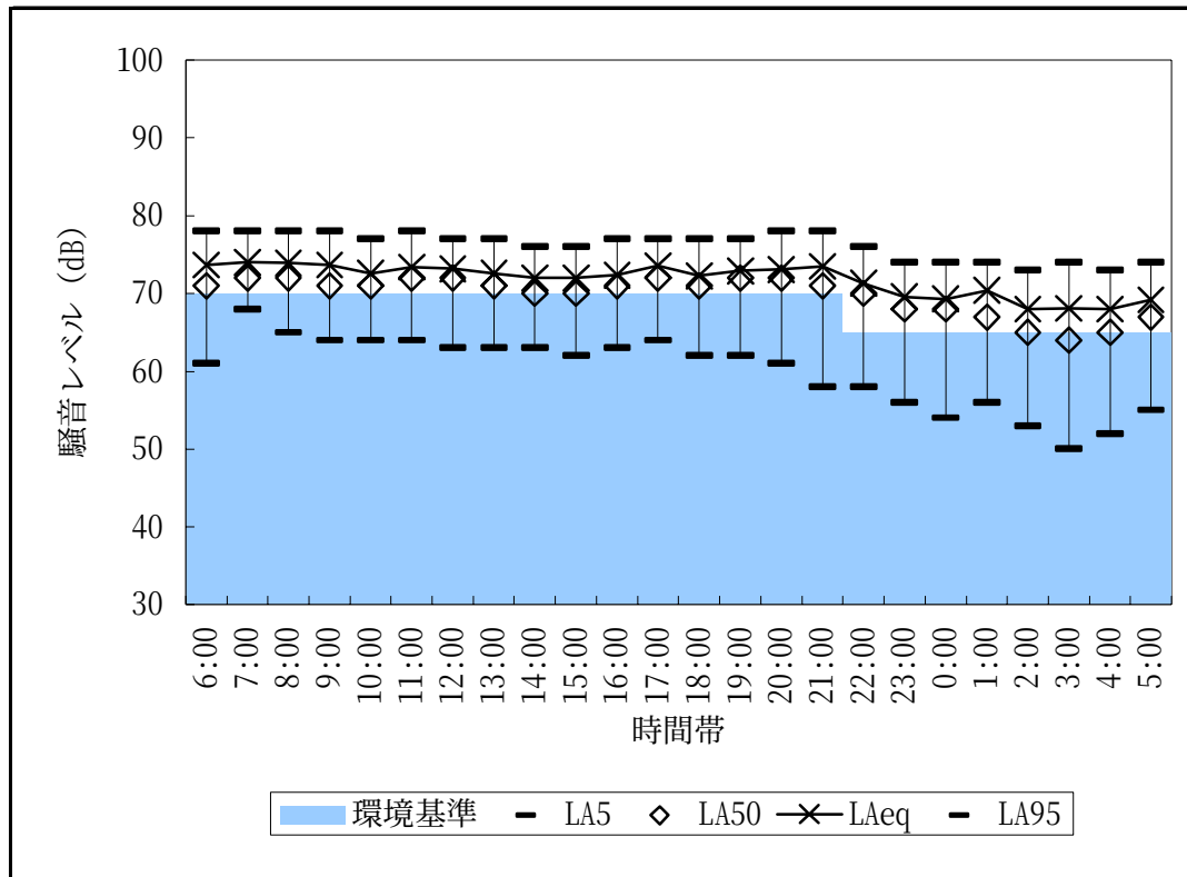
図2-3-2 騒音レベル測定結果（No.2:国道308号、センサス番号:1069、沿道）
