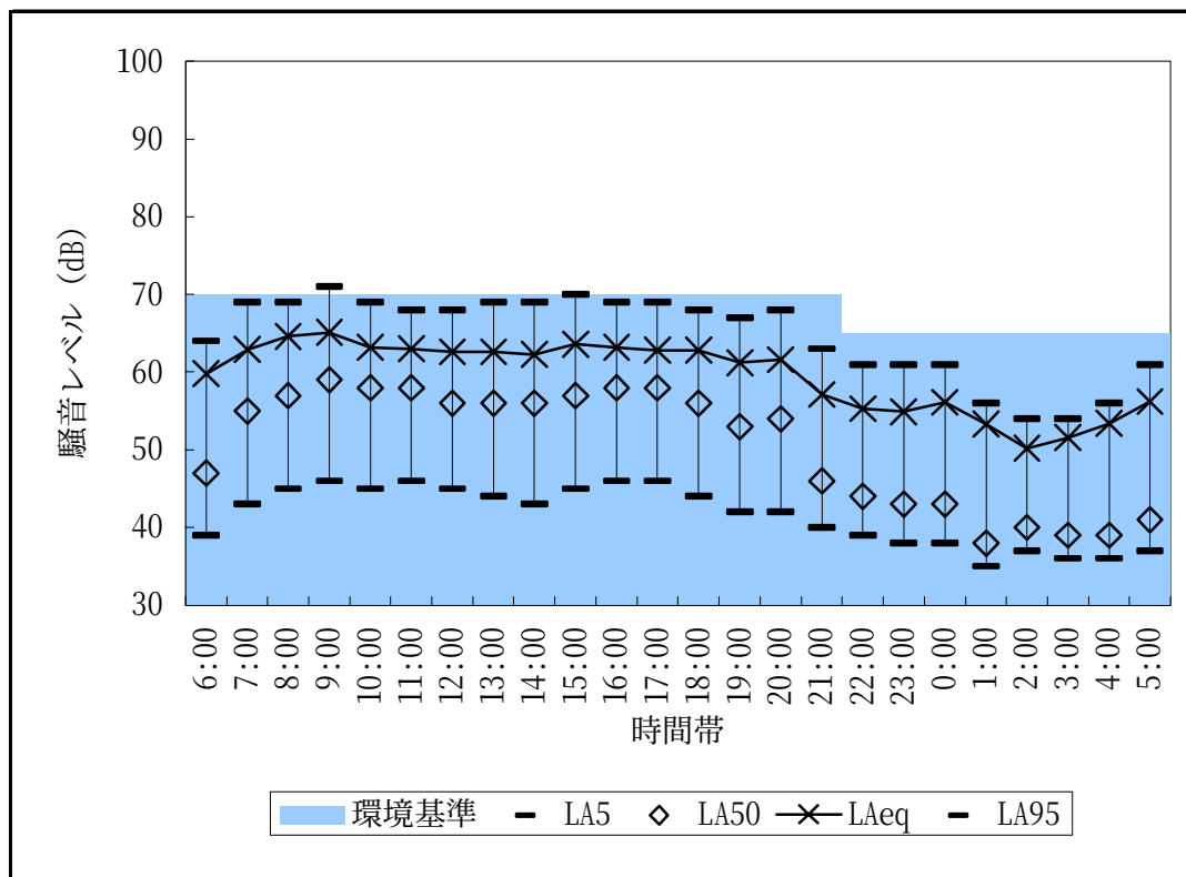
図2-3-8 騒音レベル測定結果（No.6:柳通線、沿道）
