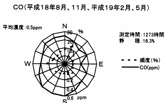
図 2-1-28 一酸化炭素の風向別濃度測定結果 (長田東内介公園)
