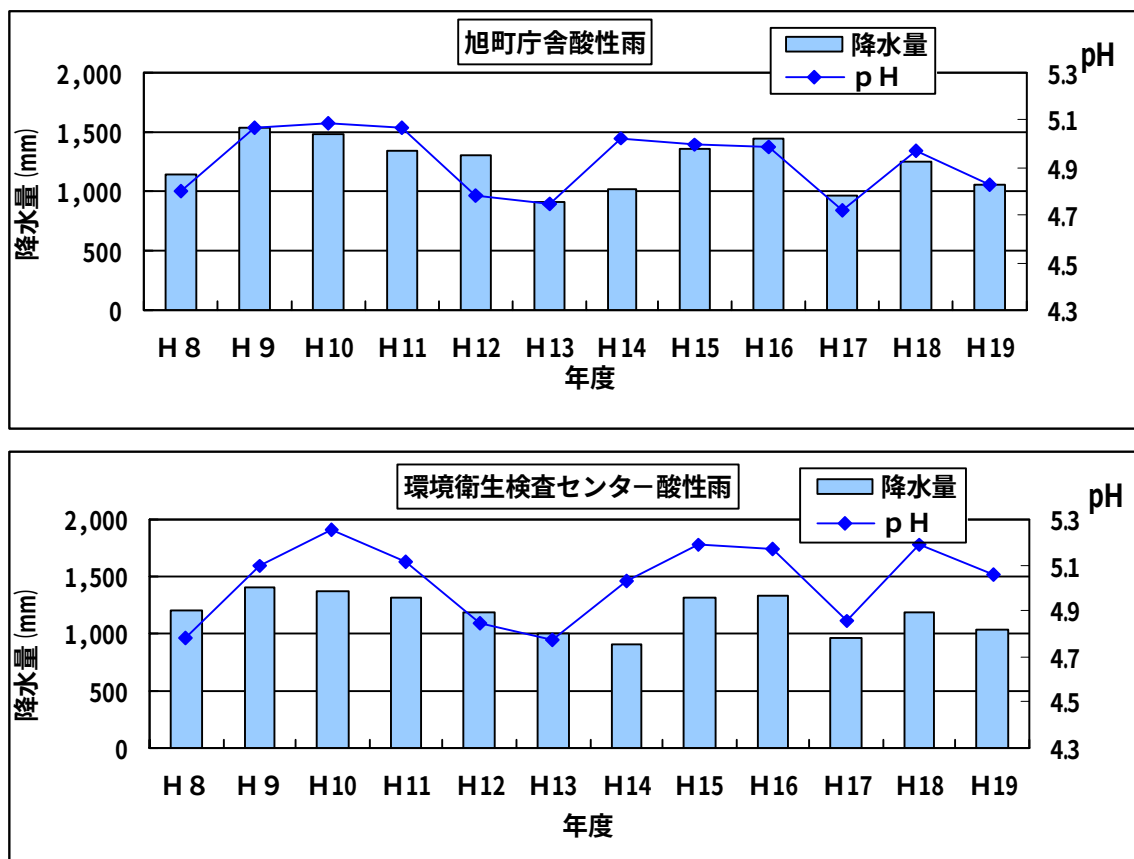
図2-1-20 酸性雨の経年変化
