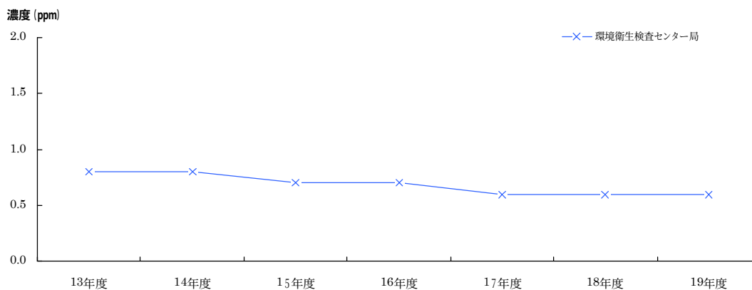
図2-1-6 一酸化炭素濃度の推移（年平均値）
