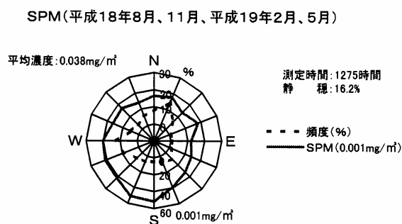
図 2-1-25 浮遊粒子状物質の風向別濃度測定結果 (長田東内介公園)
