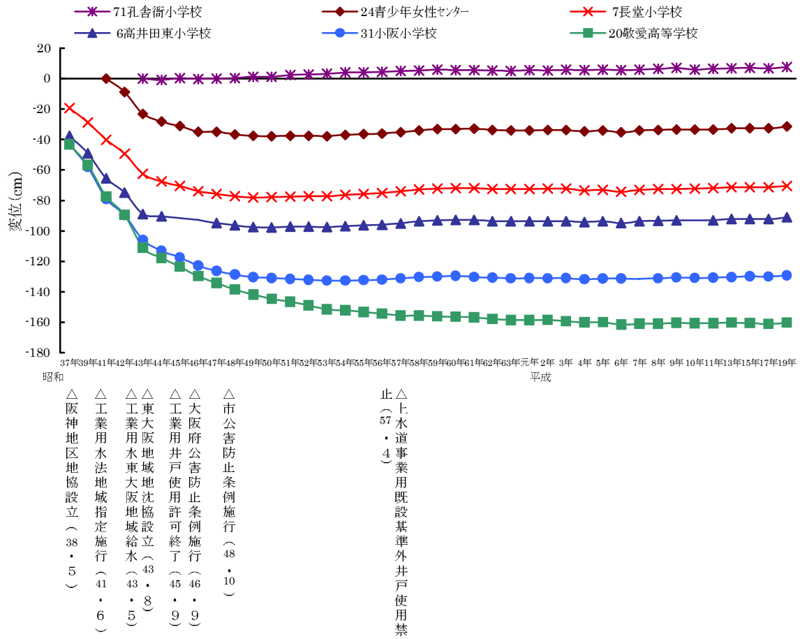
図2-5-3 代表地点における地盤変化経年図
